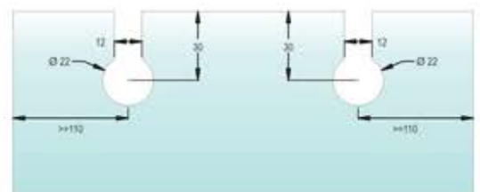
CUTOUT DETAILS OF CSL-44-A2
