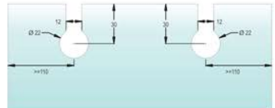
CUTOUT DETAILS OF CSL-44-A1
