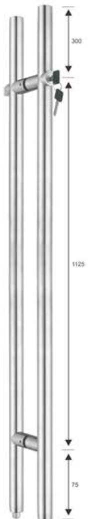
KZDHL-55 Size : 35x1500mm
